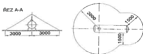
Ochranný prostor ležatého nadzemního zásobníku
