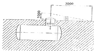
Ochranný prostor podzemního zásobníku
