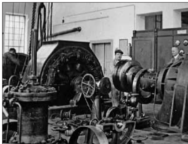
Montážní práce strojního a elektrotechnického zařízení elektrárny prováděli dělníci z plzeňské Škodovky.
